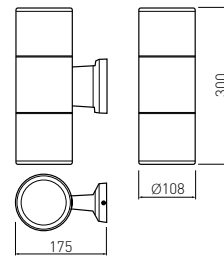
LD-BA2E27-00
