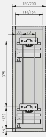
PB-K0450B0-L1
