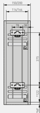
PB-K0450B0-R1
