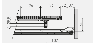
Rollschubführung / Glissière à rouleaux / Guía de rodillos
